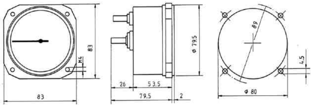
aneroid variometer 5VM
